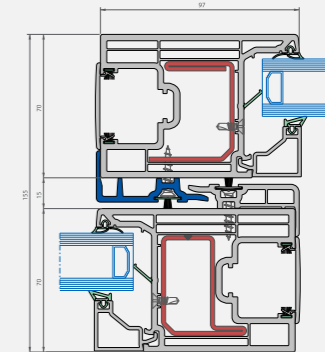
Horizontale snede
