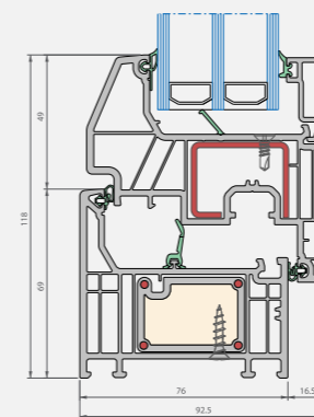
Verticale snede
