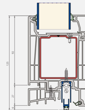
Verticale snede
