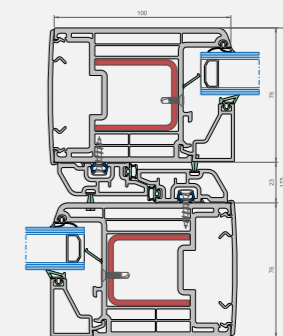
Horizontale snede
