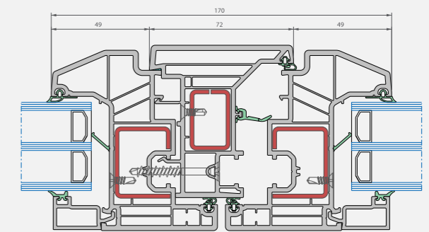
Horizontale snede
